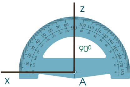
góc vuông
