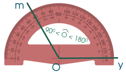
góc tù
