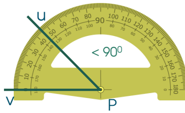
góc nhọn
